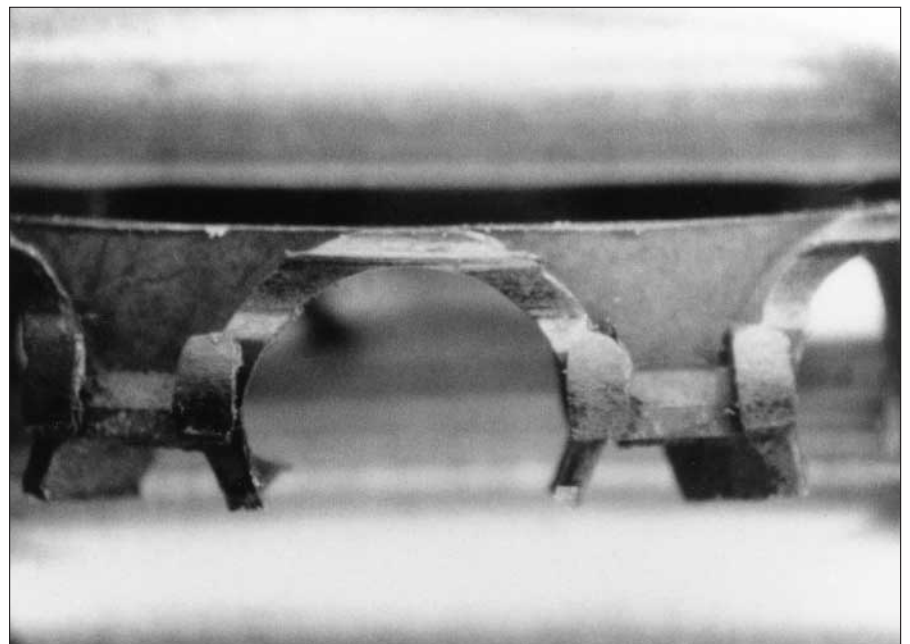
89: Desgaste en la superficie exterior de la jaula por roce con el aro exterior del rodamiento
