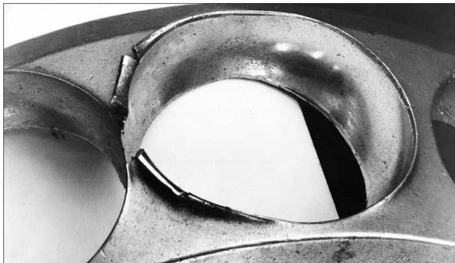
91: Debido al ladeo de los aros entre sí, se han generado fuerzas de reacción elevadas entre las bolas y la jaula, que tendrían como consecuencia la rotura de la costilla
