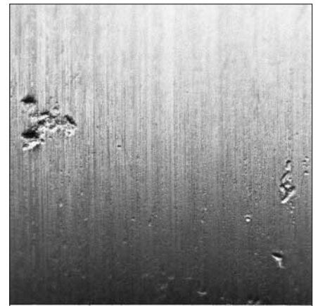
32: Indentaciones de cuerpos extraños minerales duros
