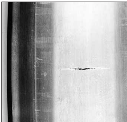
6: Daños en el aro interior detectados por medio del procedimiento de envolvente en un rodamiento oscilante de rodillos de una máquina papelera
