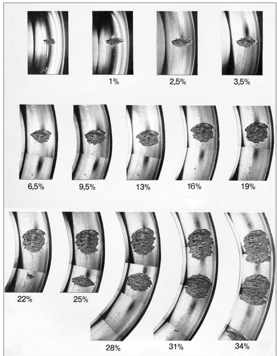
8: Evolución de daños por fatiga en el camino de rodadura del aro interior de un rodamiento de bolas de contacto angular. El intervalo de tiempo entre las revisiones desde el inicio del daño está indicado en % del tiempo de duración nominal L_{10}
