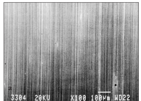
112: Fotografías de estructura superficial obtenidas con el MEB a diferentes aumentos. a: camino de rodadura intacto; b: impresiones de cuerpos extraños duros c: Daños por fatiga en su fase inicial
