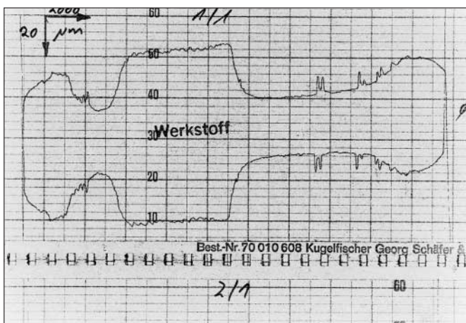
69: Registro por palpación correspondiente a la figura 68a
