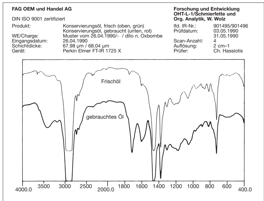
106 b: Análisis de lubricante FT-IR
