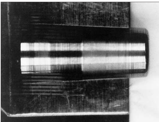
68: Formación de estrías a consecuencia de desgaste en zonas determinadas a: rodillo
