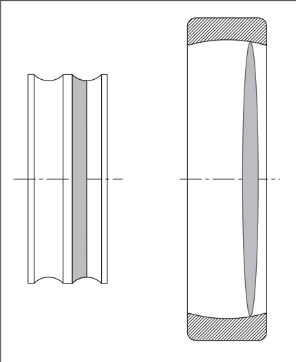
37: Configuración de las huellas de rodadura en el caso de un rodamiento oscilante de bolas con aro interior giratorio, cargado radialmente y sometido a precarga axial
