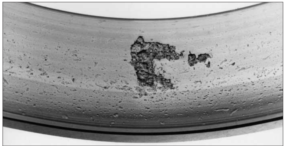
43: Deterioro por fatiga en el camino de rodadura del aro exterior de un rodamiento de rodillos cónicos
