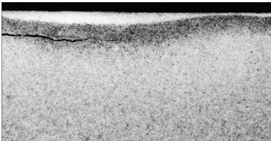
108: Sección de la zona de influencia del calor
