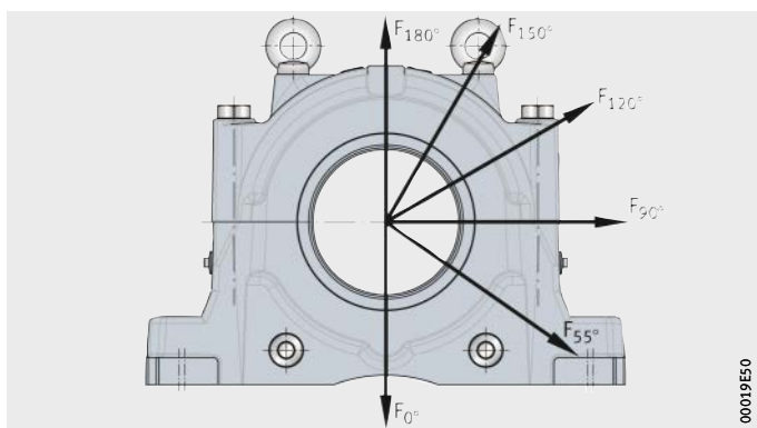
Figura 13 Direcciones de carga F para valores guía de carga de rotura de los soportes y carga máxima de los tornillos de unión
