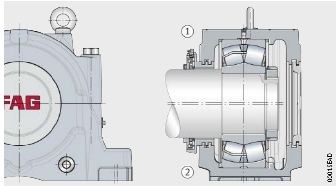
Figura 10 Soporte partido SNS para rodamientos con agujero cilíndrico (obtención de Taconite NTC y tapa NDK)
